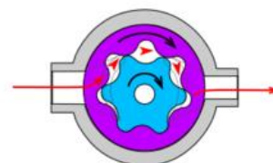
Zahnring- oder Gerolerpumpe (Füll- pumpen bei Danfoss Serie 1 und 2)
